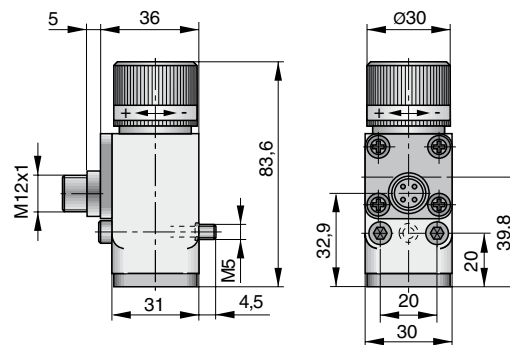
Abmessungen – Flanschausführung mit Anschluss M12x1
