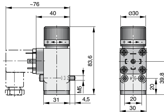
Abmessungen – Flanschausführung mit Gerätesteckdose
